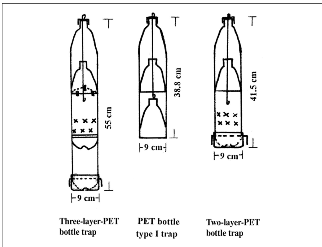
圖一 寶特瓶 I 式誘蟲器與二、三層式寶特瓶誘蟲器
