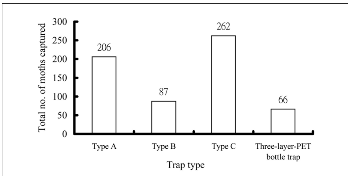
圖三 不同改良型誘蟲器於楊桃園經 6 周誘捕花姬捲葉蛾總誘蟲數之比較
